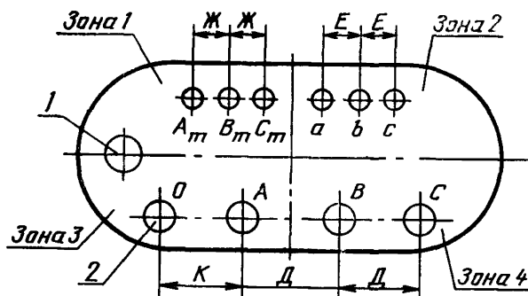
1—переключающее устройство РПН, 2—ввод нейтрали ВН
