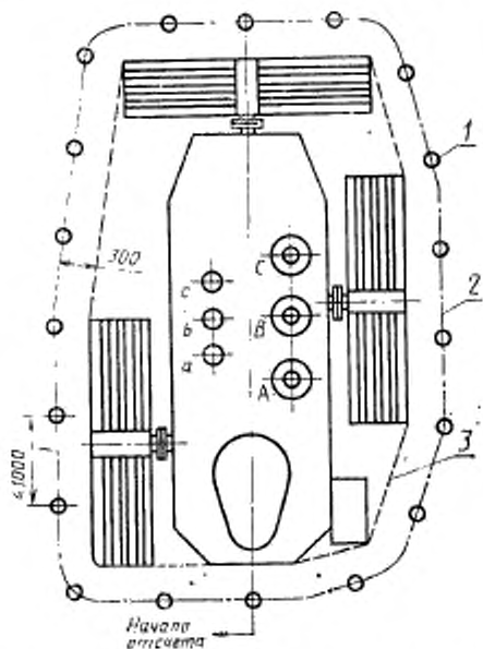
1 — микрофон; 2 — измерительная линия; 3 — излучающая поверхность
