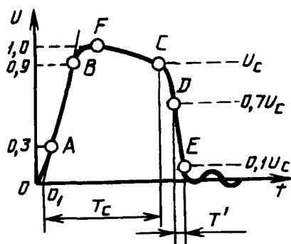
Рисунок 9 — Грозовой импульс, срезанный на спаде импульса
