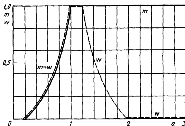
Рисунок 5 — Показатели степени m и w
