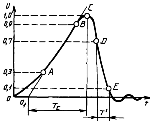
Рисунок 8 — Грозовой импульс, срезанный на фронте
