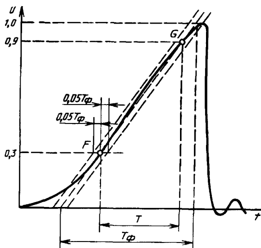
Рисунок 10 — Линейно нарастающий импульс
