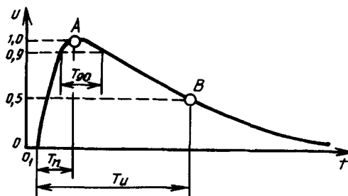
Рисунок 13 — Аperiodический коммутационный импульс
