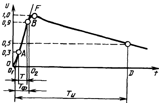
Рисунок 7 — Полный грозовой импульс
