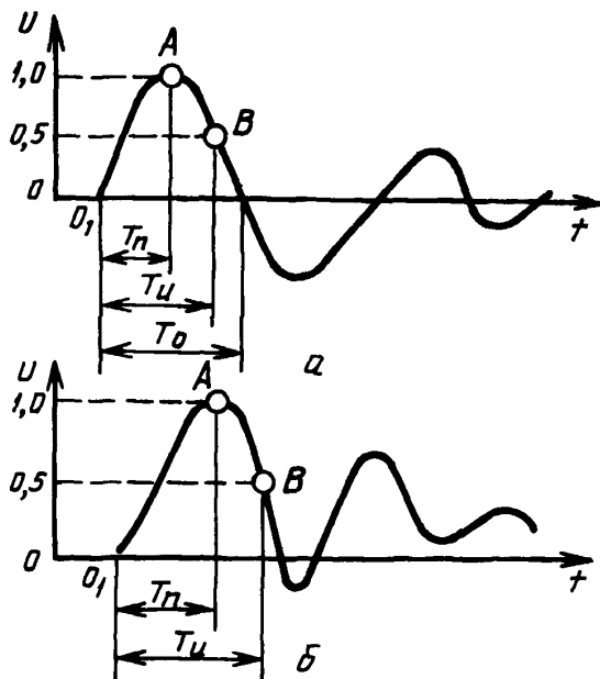
Рисунок 14 — Колебательный коммутационный импульс
