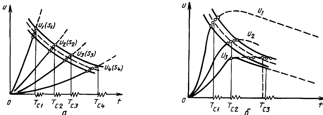
Рисунок 12 — Вольт-секундные характеристики
