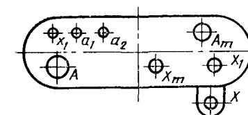
а) автотрансформатор АОДЦТН-333000/750/330
