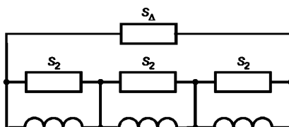
Рисунок 1 — Схема подключения фазных нагрузок
