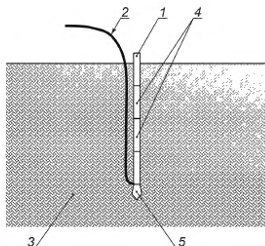
1 — короткий самый верхний отрезок заглубляемого стержня; 2 — проводник заземлителя; 3 — грунт; 4 — отрезки заглубляемого стержня; 5 — стальное острие
