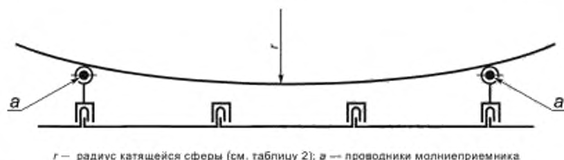
Рисунок Е.26 — Конструкция сети молниеприемников на крыше с проводящим покрытием, где пробы покрытия не допустим
