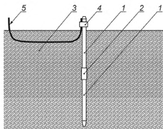
1 — удлиняемый вертикальный заземлитель; 2 — муфта заземлителя; 3 — грунт; 4 — зажим на вертикальном заземлителе; 5 — заземляющий проводник
