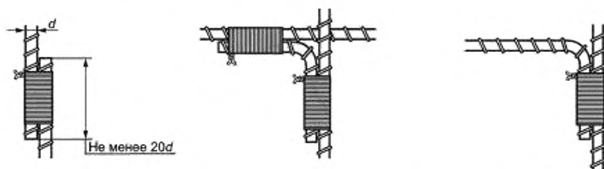
с) Соединения с помощью вязки, применяемые в условиях тока молнии и целей ЭМС
