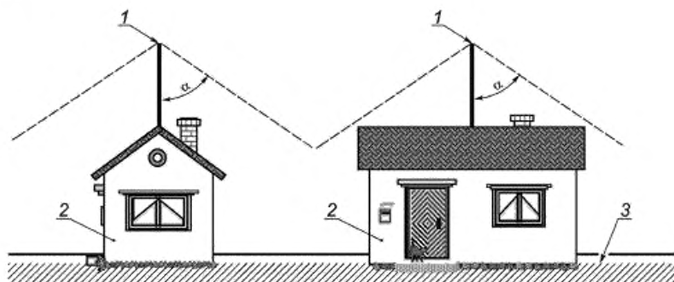
а) Пример использования одного стержневого молниевывода
