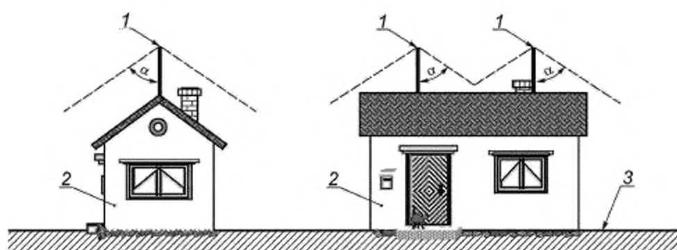
б) Пример использования двух стержневых молниевыводов
