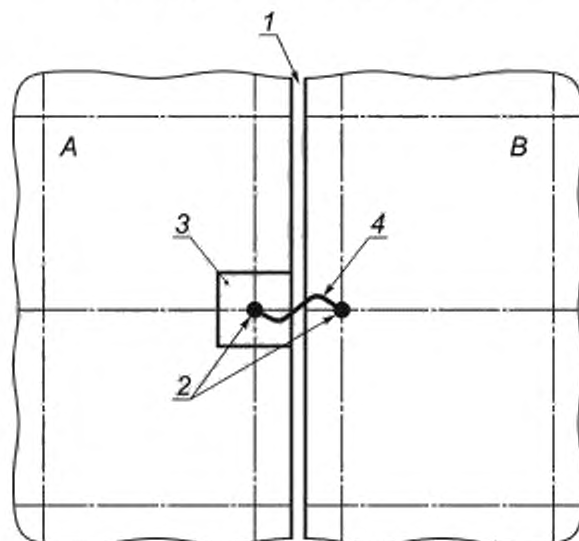
1 — компенсационный зазор, 2 — сварное соединение; 3 — углубление; 4 — гибкий проводник уравнивания потенциалов, А — железобетонный элемент 1; В — железобетонный элемент 2
