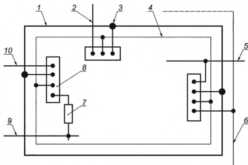
1 — стальная арматура внешней железобетонной стены и фундамента; 2 — другой заземлитель; 3 — разъем для уравнивания потенциалов; 4 — внутренний кольцевой проводник; 5 — присоединение к внешней проводящей части, например водопроводной трубе; 6 — кольцевой заземлитель, заземляющее устройство конфигурации В; 7 — устройство защиты от перенапряжений; 8 — шина уравнивания потенциалов; 9 — линия электроснабжения или линия связи; 10 — заземляющее устройство конфигурации А к дополнительному заземлителю
