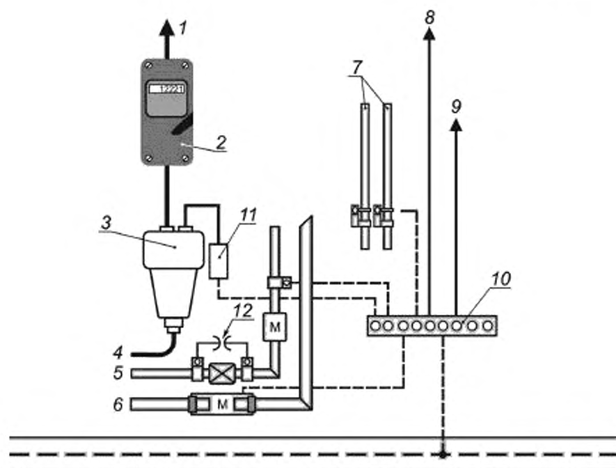
1 — ввод к потребителю электроэнергии; 2 — счетчик электроэнергии; 3 — вводная клеммная коробка; 4 — ввод электроэнергии от питающей сети; 5 — газ; 6 — вода; 7 — система центрального отопления; 8 — к электронным устройствам; 9 — к экрану кабеля антенны; 10 — шина уравнивания потенциалов; 11 — устройство защиты от перенапряжений; 12 — разделительный искровой разрядник; М — счетчик
