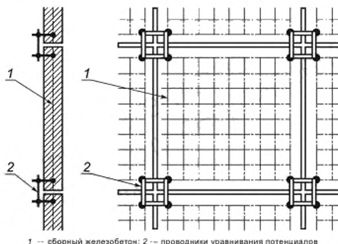
1 — сборный железобетон; 2 — проводники уравнивания потенциалов
