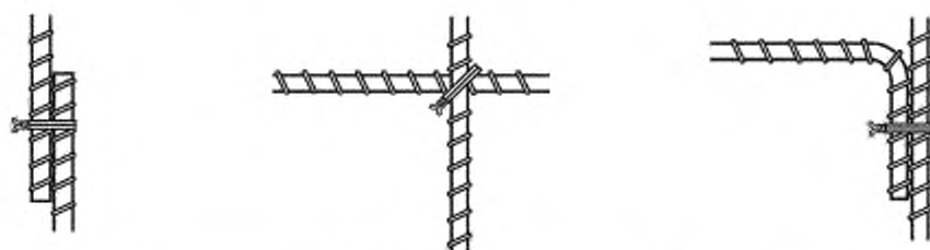
д) Соединения с помощью вязки, пригодные только для целей ЭМС
