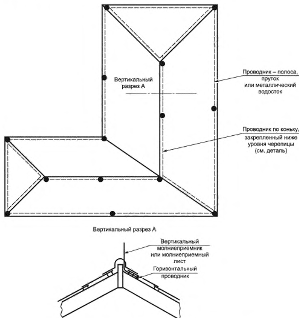
Рисунок Е.23 — Молниеприемник и скрытые проводники для сооружений высотой менее 20 м со скатыми крышами
