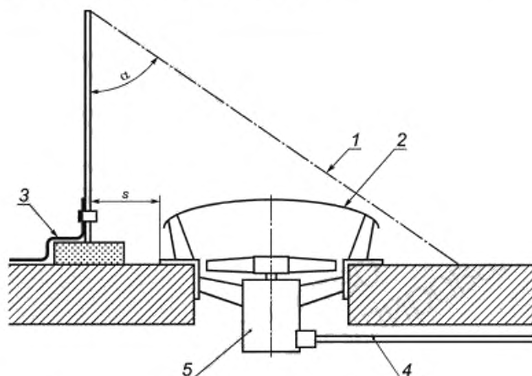
1 — зона защиты в виде конуса; 2 — металлическая конструкция на крыше; 3 — горизонтальный проводник молниеприемника; 4 — линия электропитания установки, по возможности расположенная в проводящем экране; 5 — электрическое оборудование; s — разделительное расстояние в соответствии с 6.3; \alpha — защитный угол в соответствии с таблицей 2
