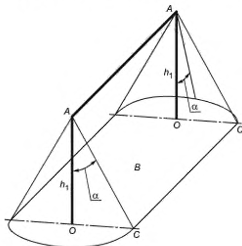
Рисунок А.3 — Объем, защищаемый тросовым молниеприемником
