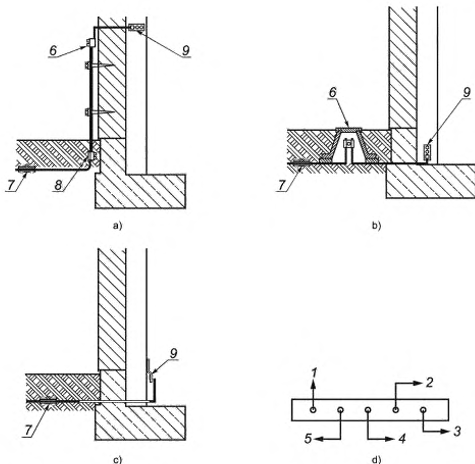
Вариант 1 — Испытательный зажим на стене
