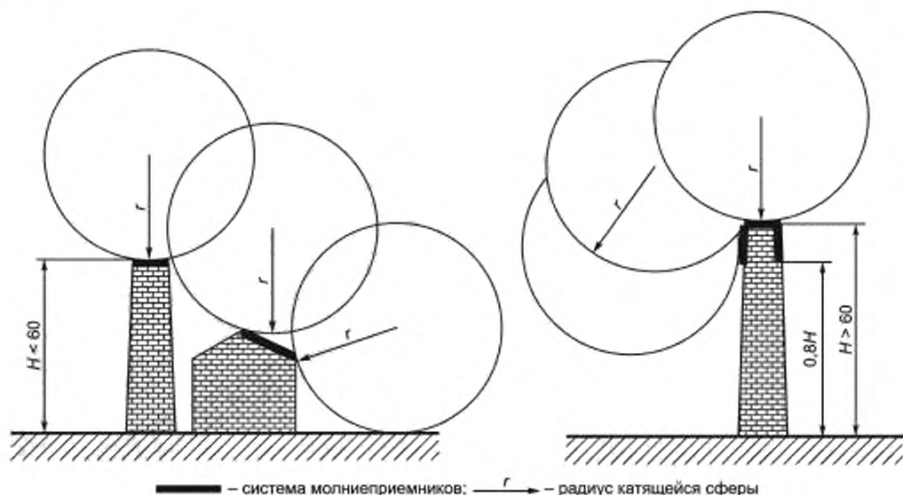
Рисунок А.6 — Проектирование системы молниеприемников по методу катящейся сферы
