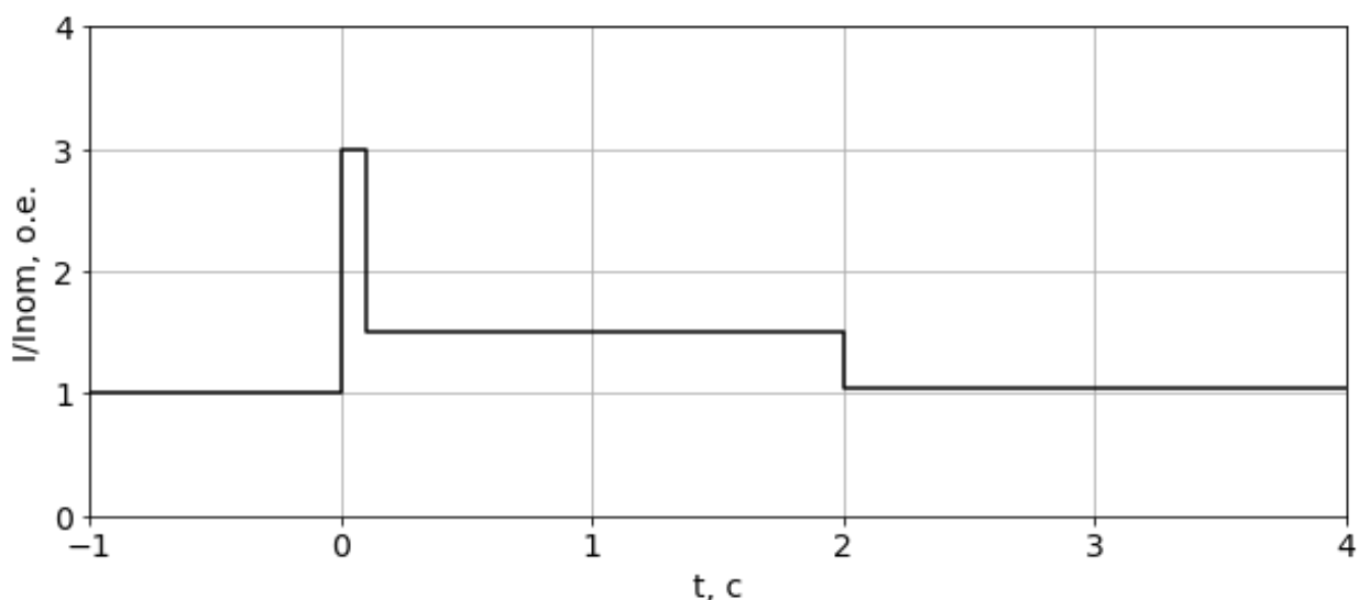
Рис. 11.1. Требования к выходному току DC/DC конвертора в режимах коротких замыканий и пусковых токов электроприемников.
