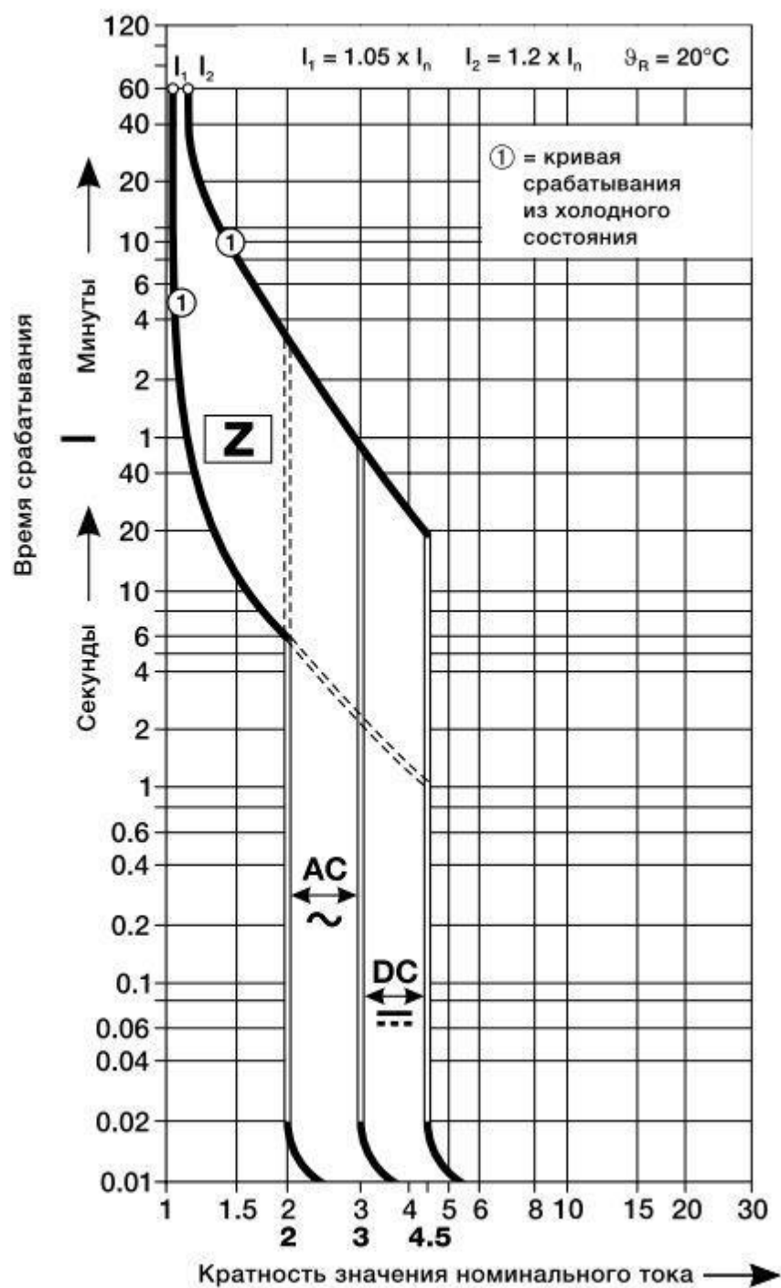
Рис. Д.4. Время-токовая защитная характеристика типа Z.
