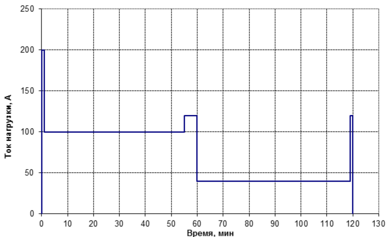
Рис. А.4. Диаграмма нагрузки СОПТ
